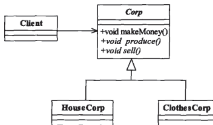
图29-1 盈利模式的类图
