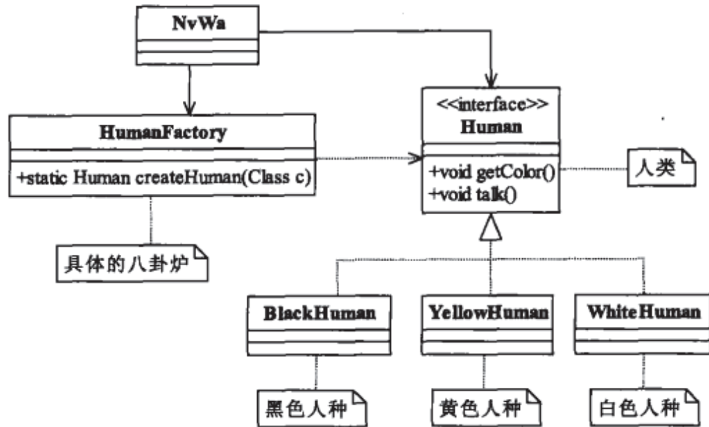
图8-3 简单工厂模式类图
