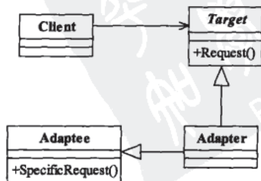
图19-4 适配器模式通用类图
