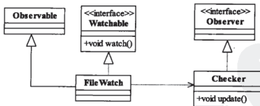
图38-5 XML文件监控类图
