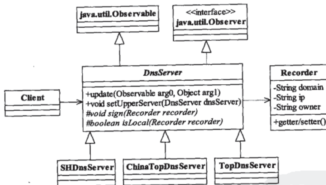
图32-10 触发链模式实现DNS解析的类图
