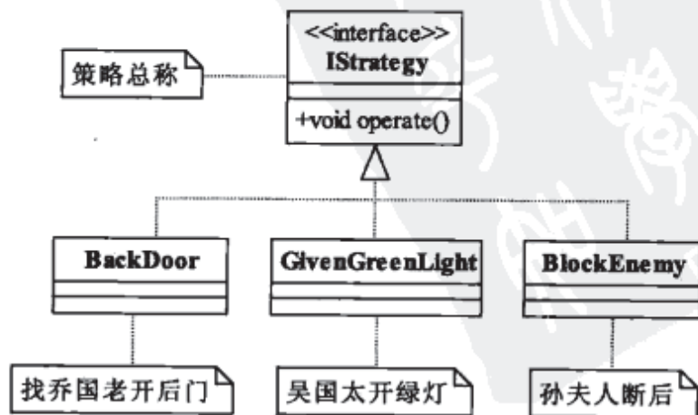
图18-1 三个策略类图
