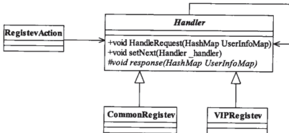
图16-5 用户注册类图
