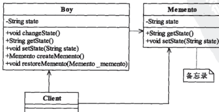
图24-2 完善后的男孩状态类图
