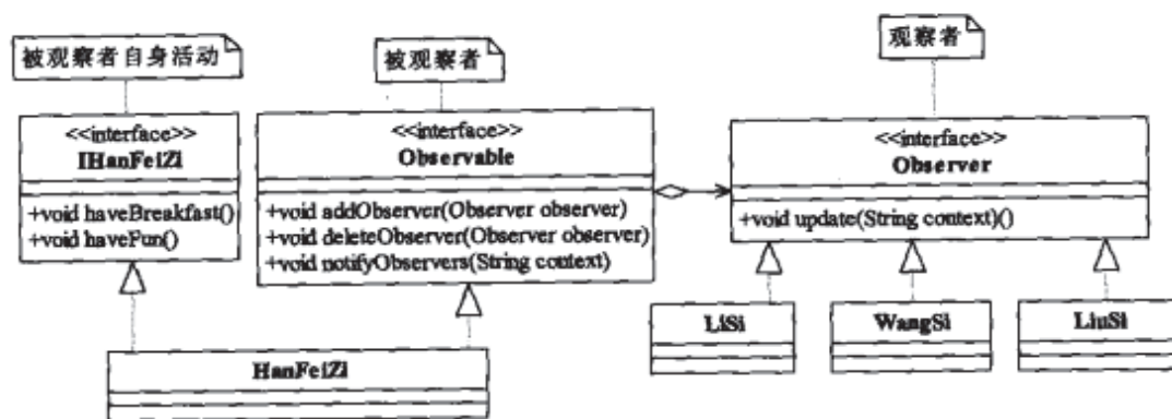
图22-4 改进后的观察者和被观察者
