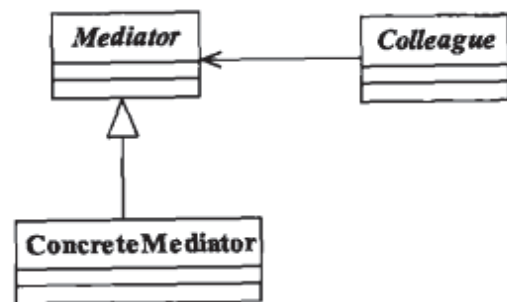
图14-7 中介者模式通用类图
