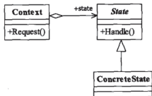
图26-5 状态模式通用类图
