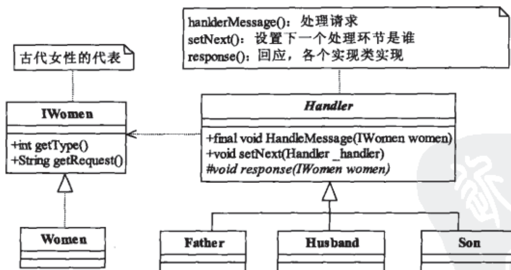
图16-3 顺序处理的类图
