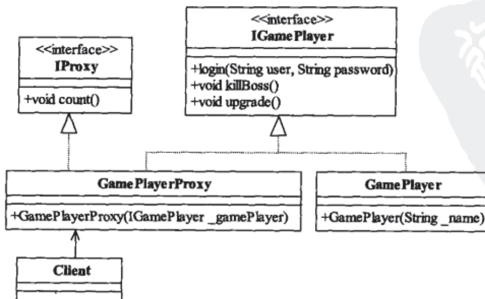
图12-6 代理类的个性
