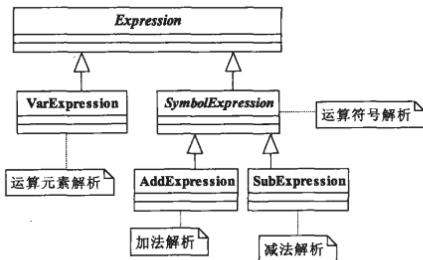
图27-1 初步分析加减法类图
