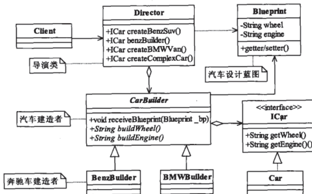
图30-4 建造者模式建造车辆
