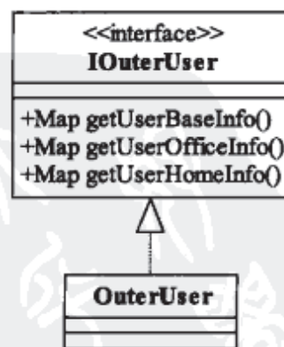
图19-2 劳动服务公司的人员信息类图
