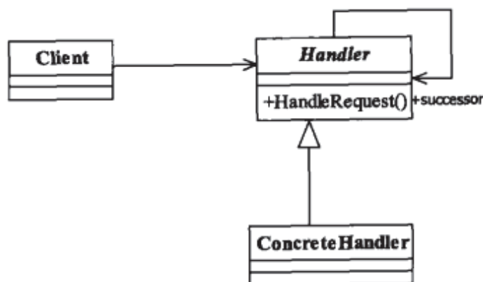
图16-4 责任链模式通用类图
