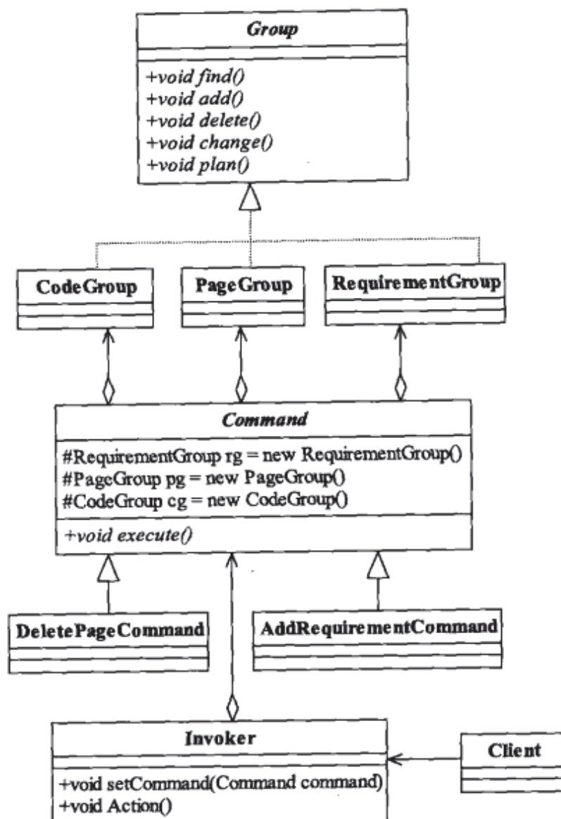
图15-3 完美的类图
