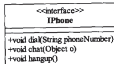
图1-4 电话类图
