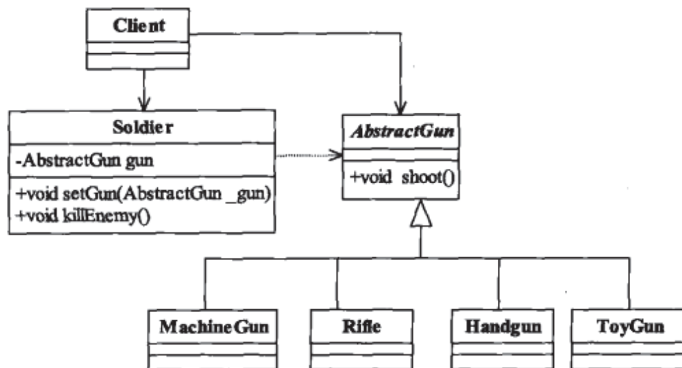
图2-2 枪支类图
