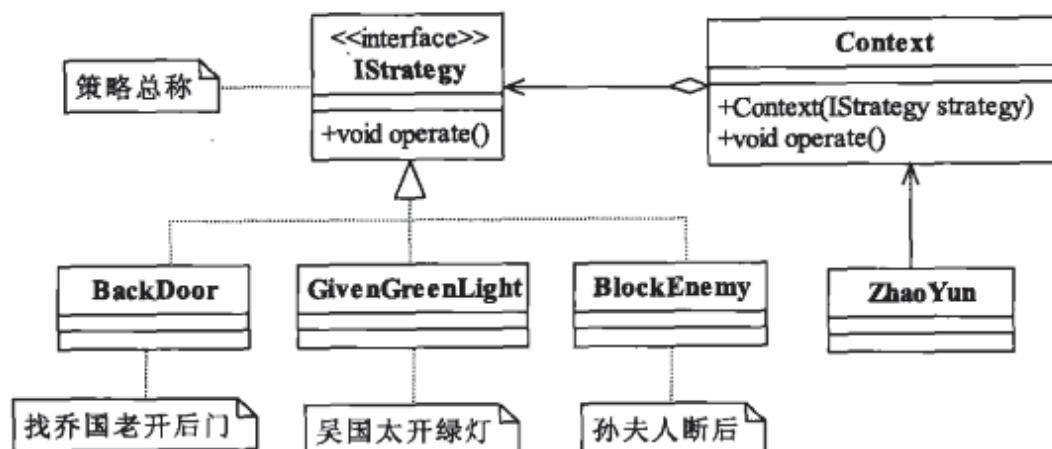
图18-2 完整类图
