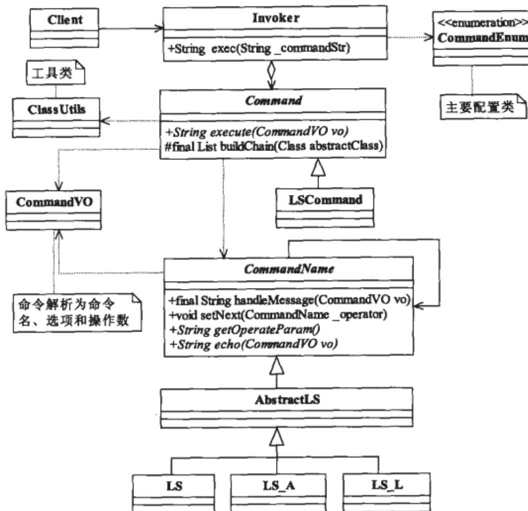
图34-4 完整类图
