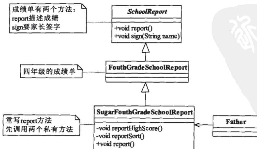
图17-3 修饰成绩单
