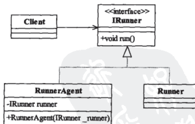
图31-1 运动员跑步
