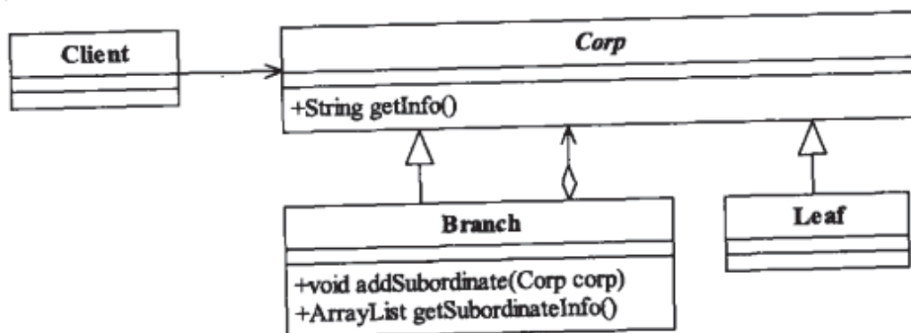
图21-5 精简的类图
