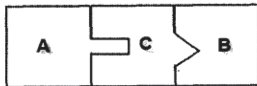
图19-7 完美组合
