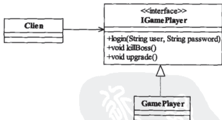
图12-1 游戏过程
