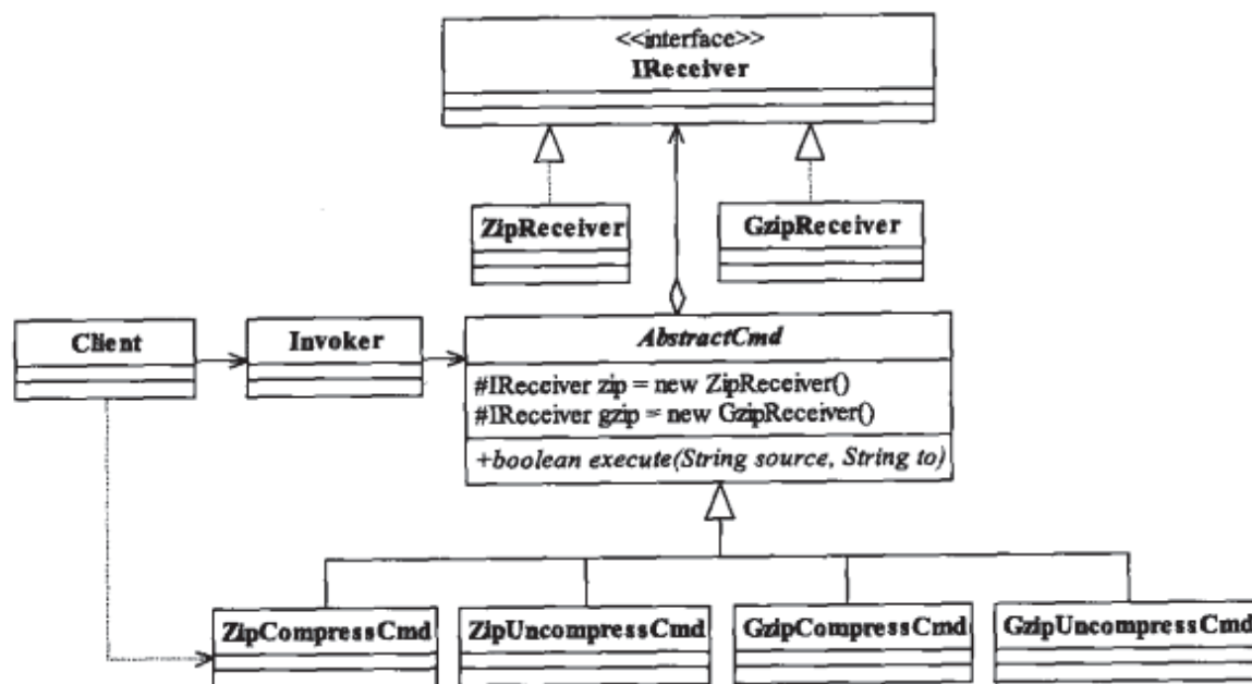
图32-2 命令模式实现压缩算法的类图
