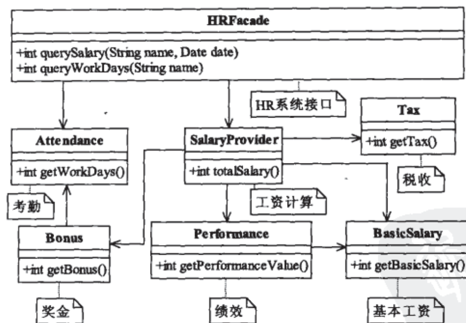
图33-5 HR系统的类图
