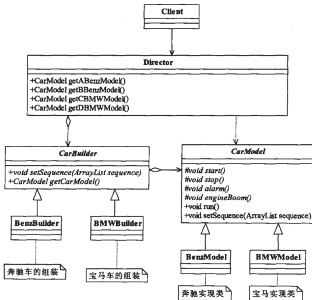
图11-3 完整汽车模型类图
