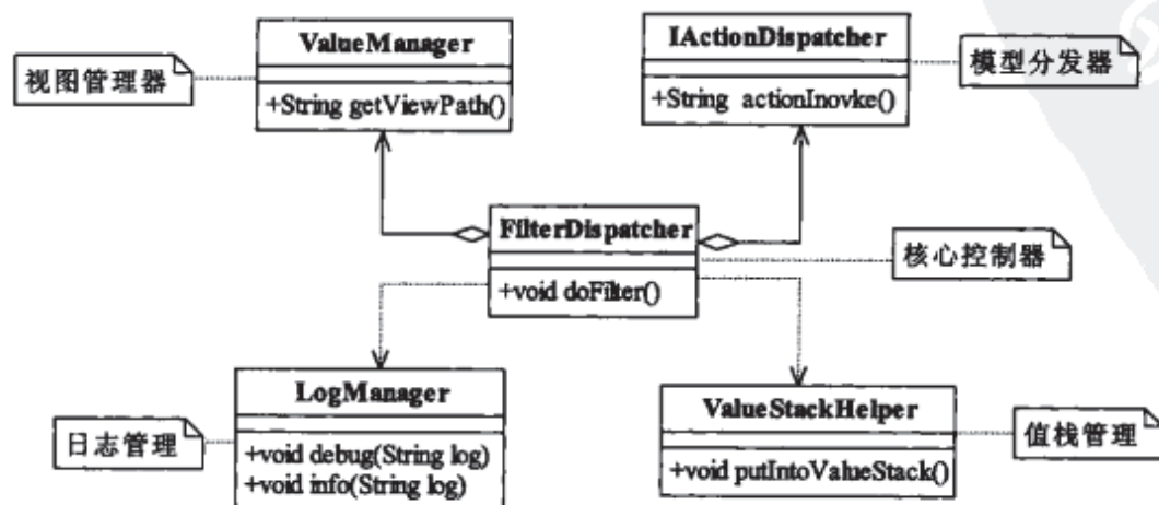
图38-4 核心控制器类图
