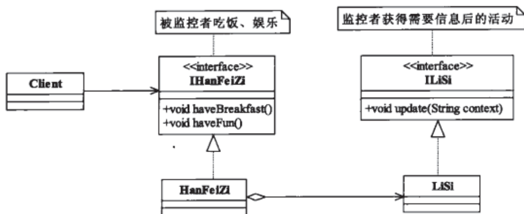
图22-3 通过聚集方式监控
