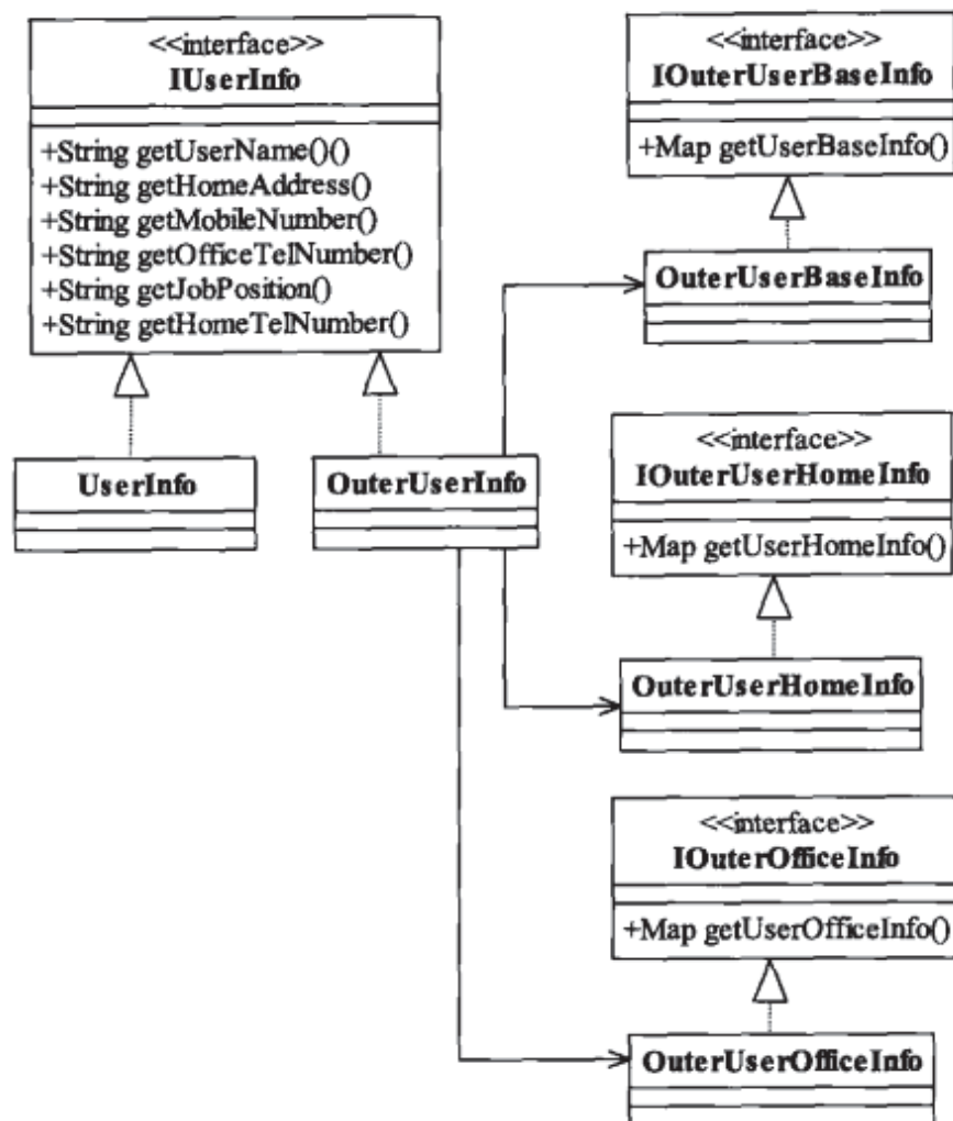
图19-8 拆分接口后的类图
