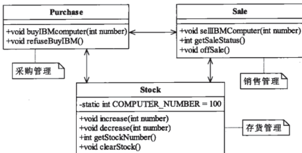
图14-2 简单的进销存类图
