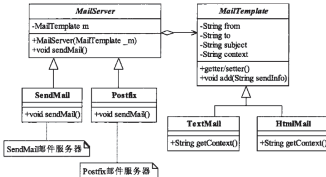
图33-3 桥梁模式实现邮件发送的类图
