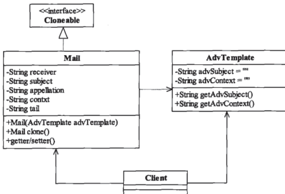
图13-2 修改后的发送电子账单类图
