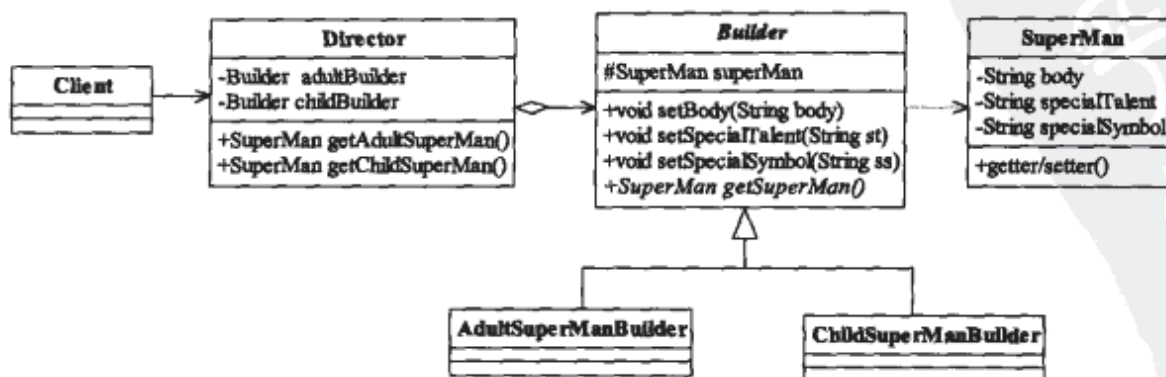
图30-2 按建造者模式生产超人
