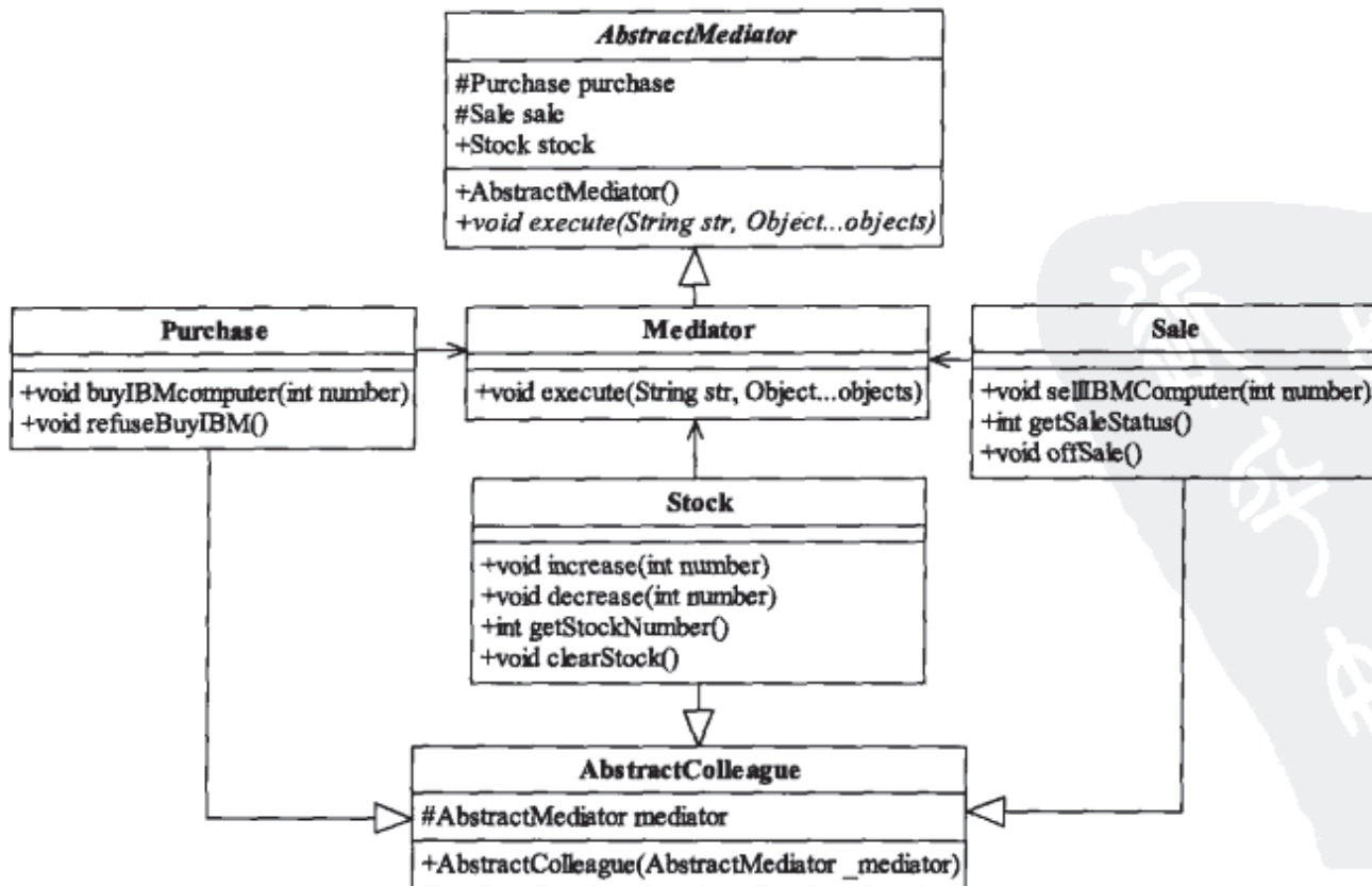
图14-6 修改后的进销存类图
