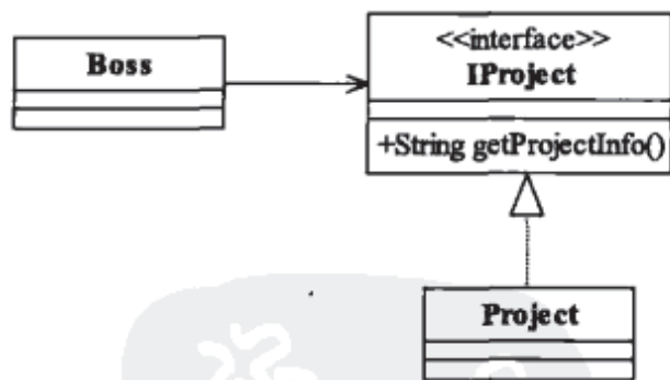
图20-1 项目信息类图
