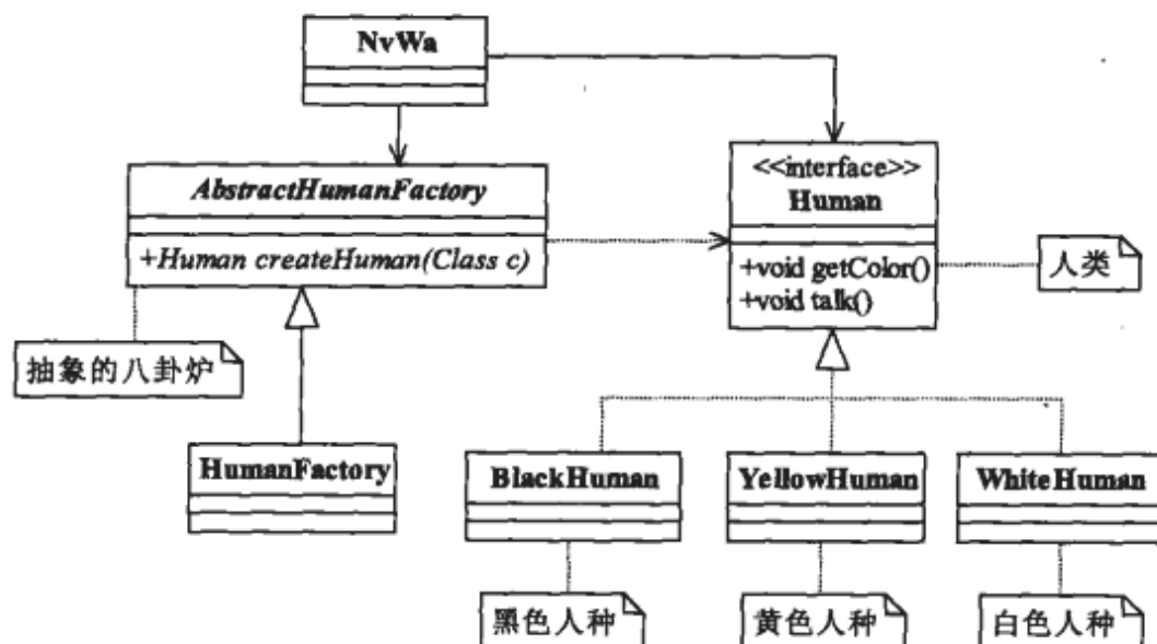
图8-1 女娲造人类图
