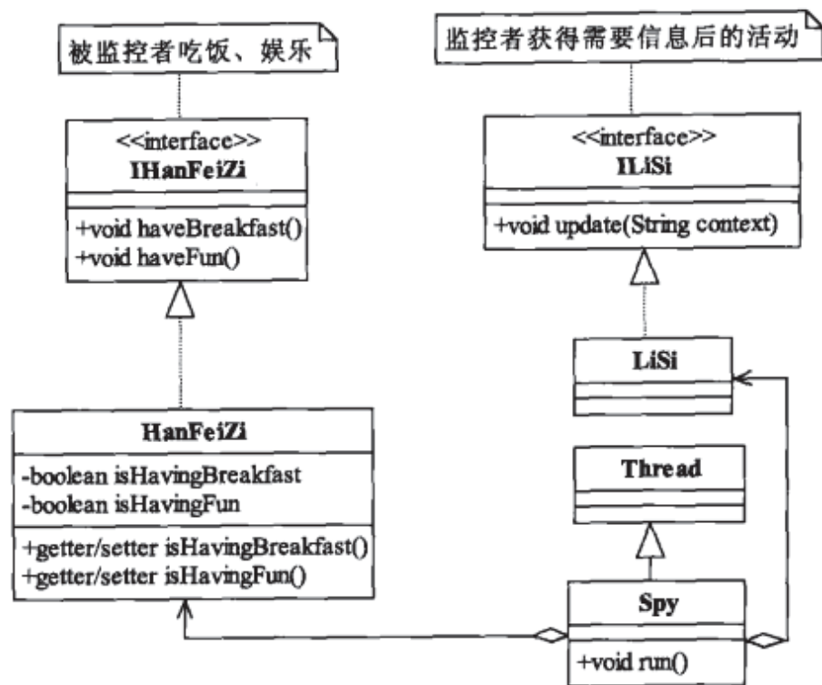
图22-2 通过后台线程监控
