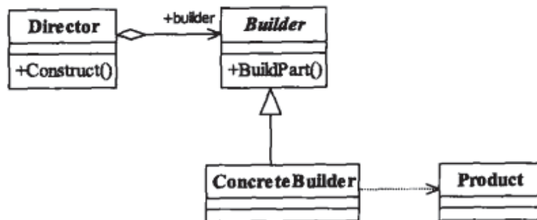
图11-4 建造者模式通用类图
