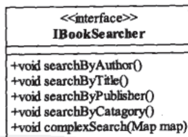
图4-4 图书查询类图
