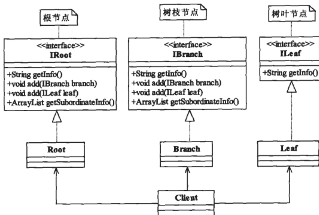
图21-2 最容易想到的组织架构类图
