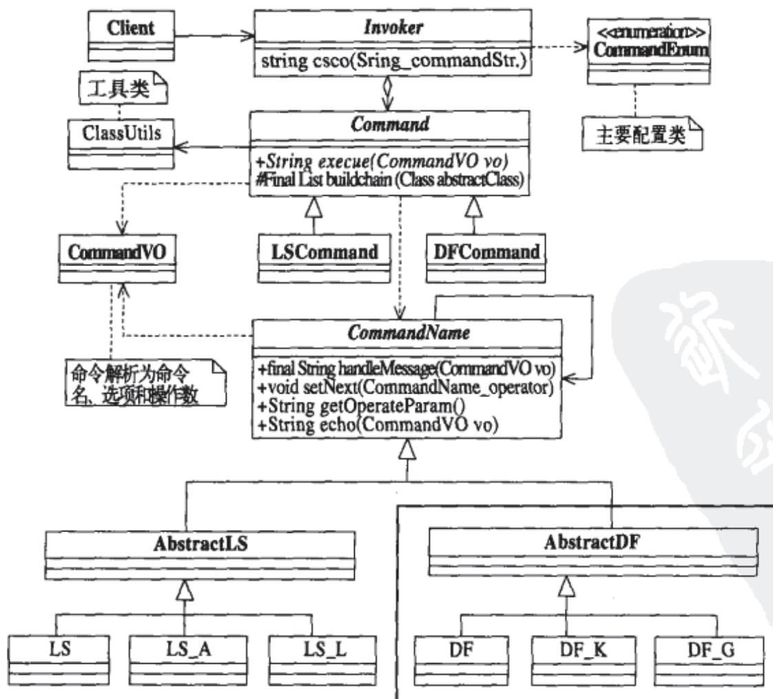
图34-5 扩展df命令后的类图
