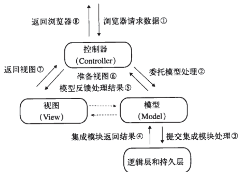
图38-2 MVC框架的逻辑流
