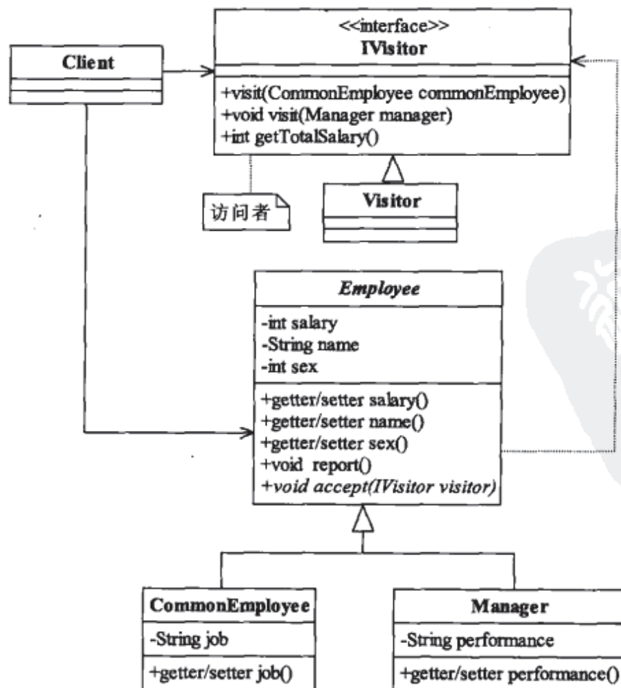
图25-6 统计功能的访问者模式
