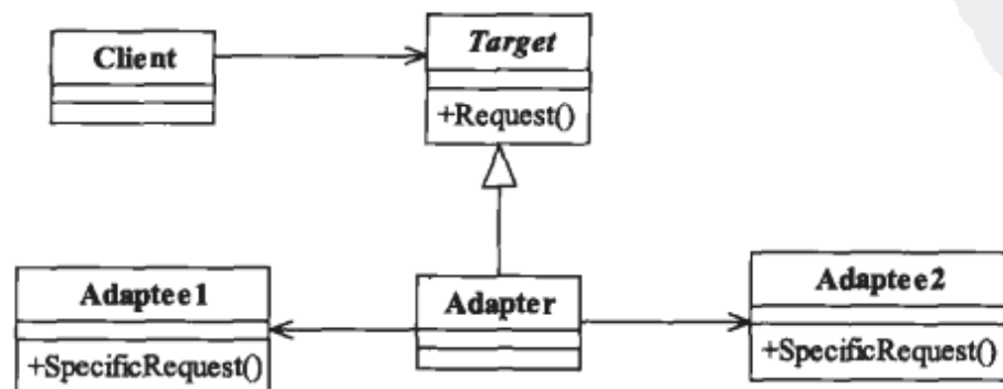
图19-9 对象适配器类图
