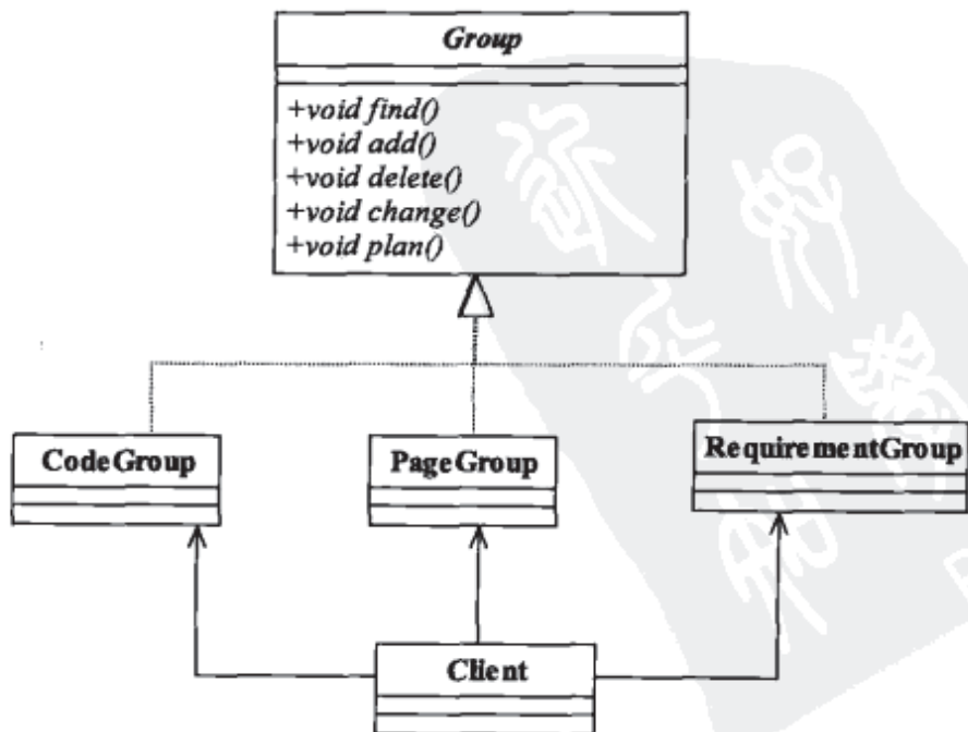
图15-1 旅行社项目开发过程类图
