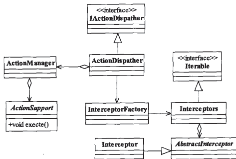
图38-6 模型管理器类图
