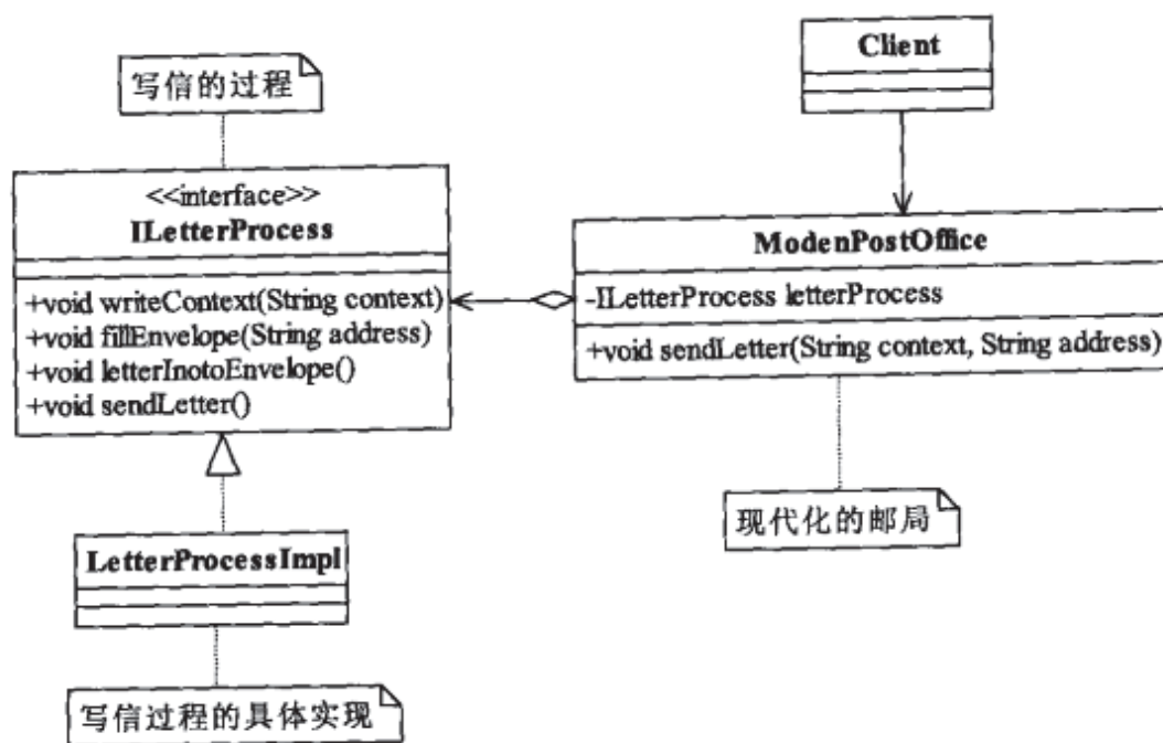
图23-2 增加现代化邮局的类图
