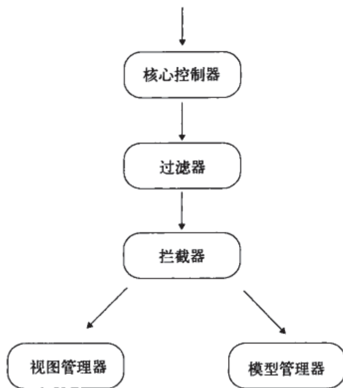
图38-3 MVC系统架构
