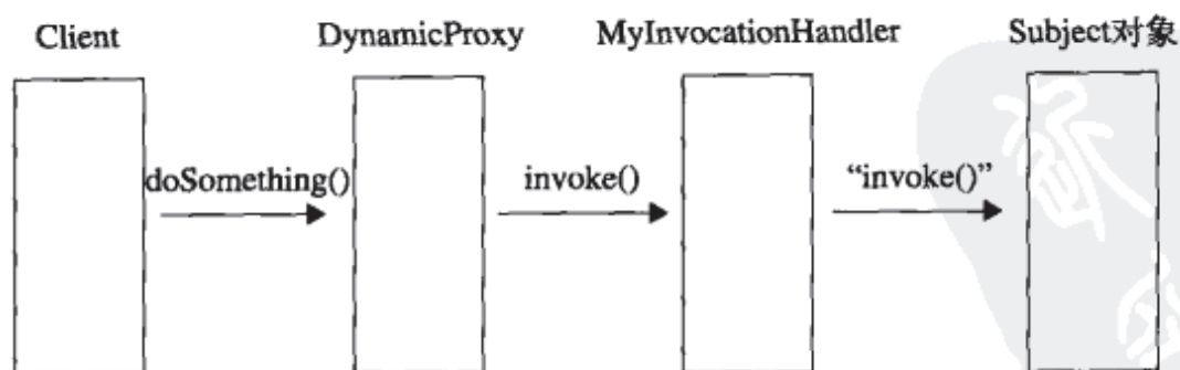
图12-9 动态代理调用过程示意图
