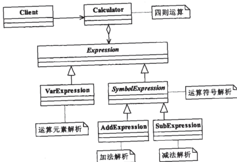
图27-2 优化后加减法类图
