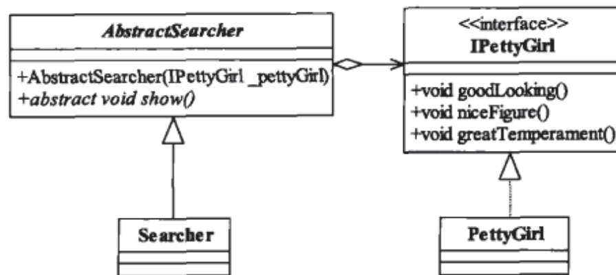
图4-1 星探寻找美女的类图
