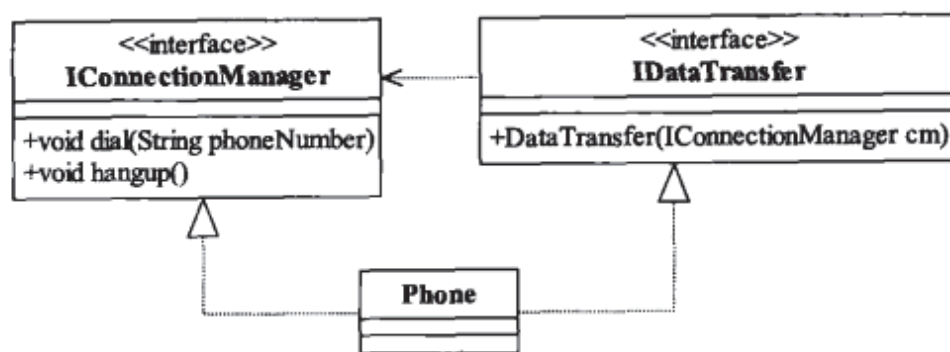
图1-6 简洁清晰、职责分明的电话类图
