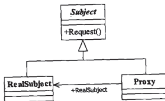
图12-3 代理模式的通用类图
