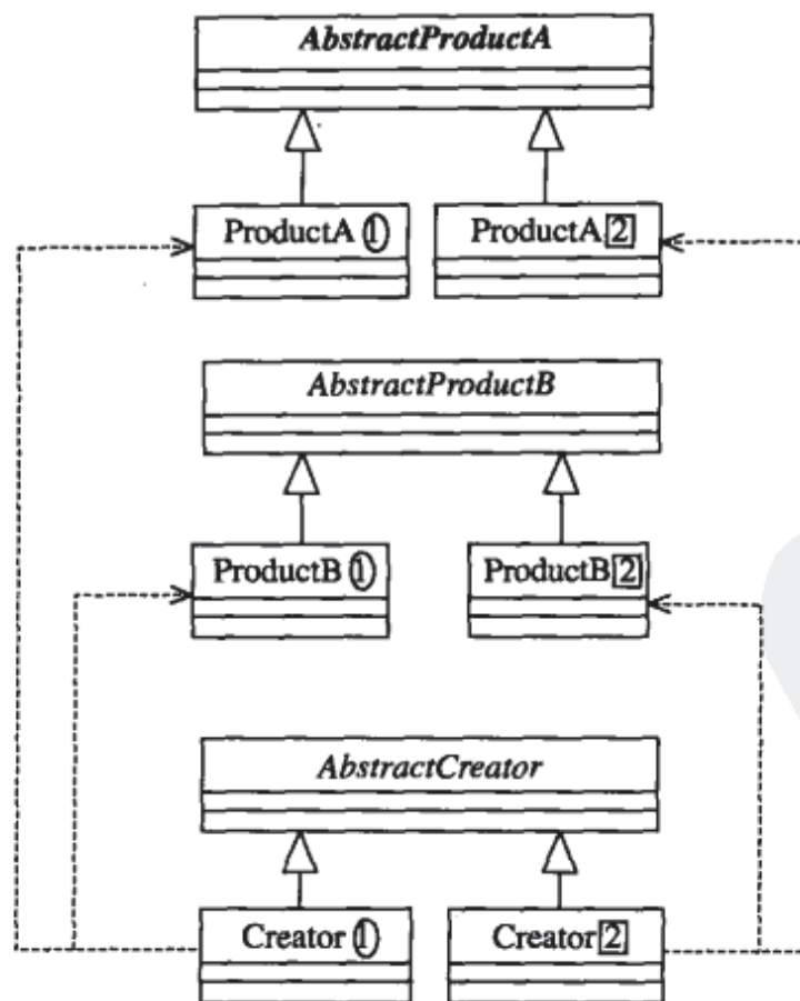
图9-4 抽象工厂模式的通用源码类图
