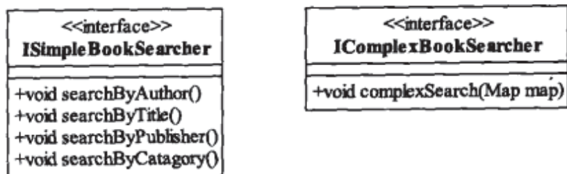
图4-5 修改后的图书查询类图
