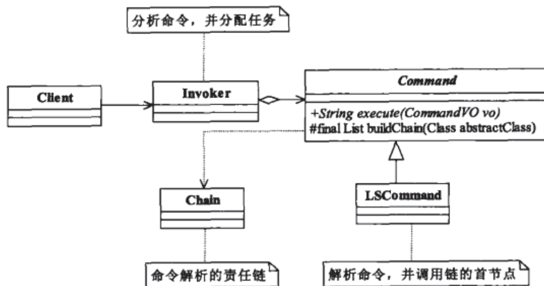
图34-3 命令传递类图
