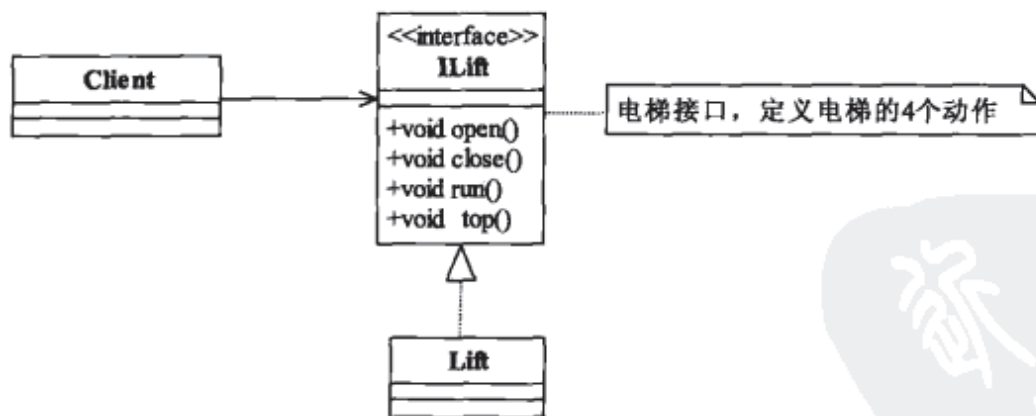
图26-1 电梯的类图
