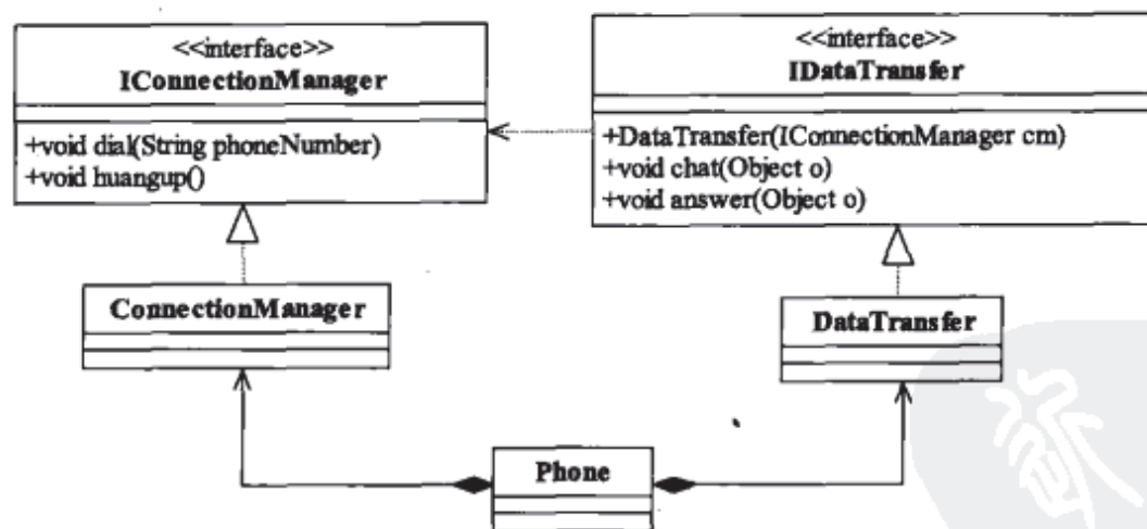
图4-3 电话类图
