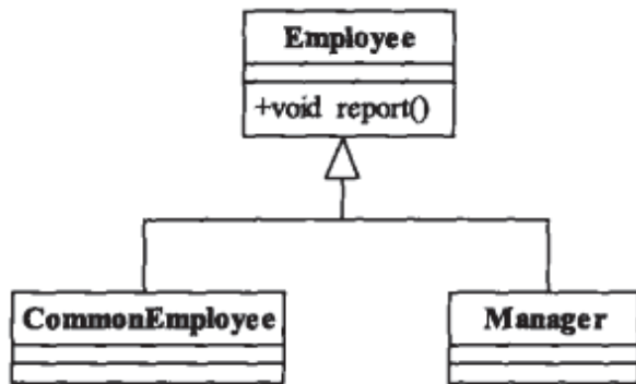
图25-2 简化类图
