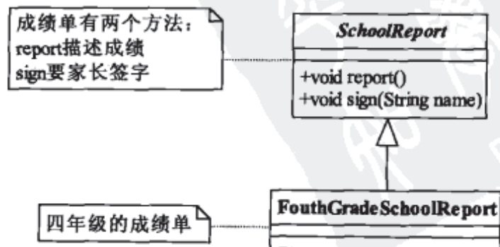
图17-1 成绩单类图
