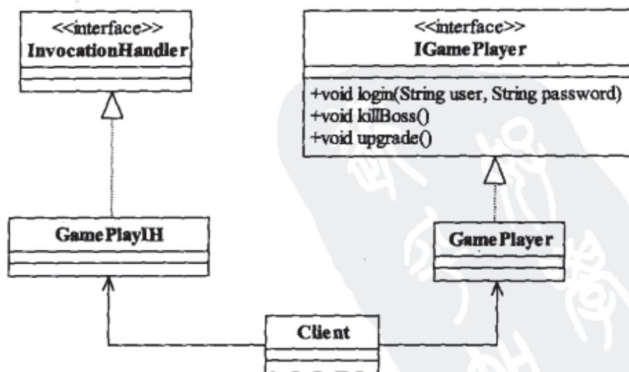
图12-7 动态代理
