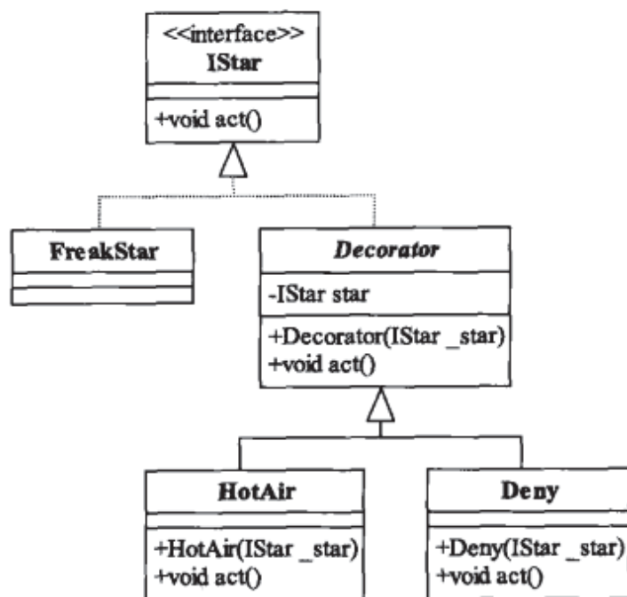
图33-7 演技修饰
