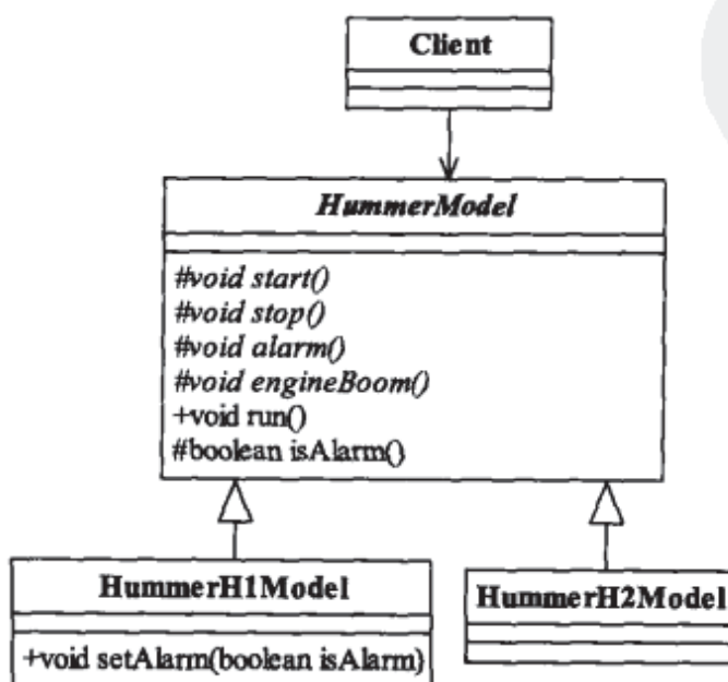
图10-4 扩展悍马车模类图
