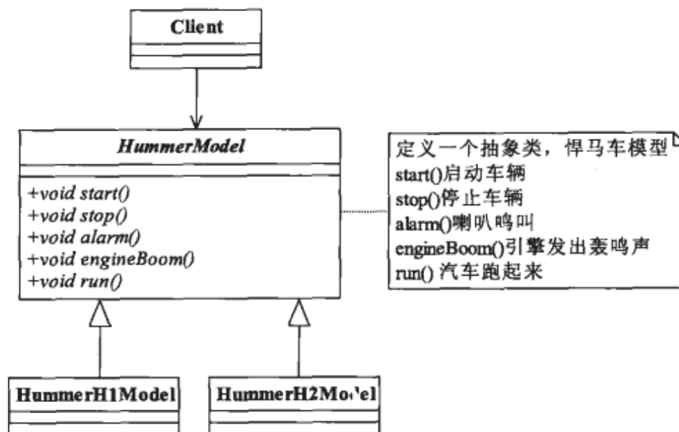
图10-1 悍马车模型最一般的类图
