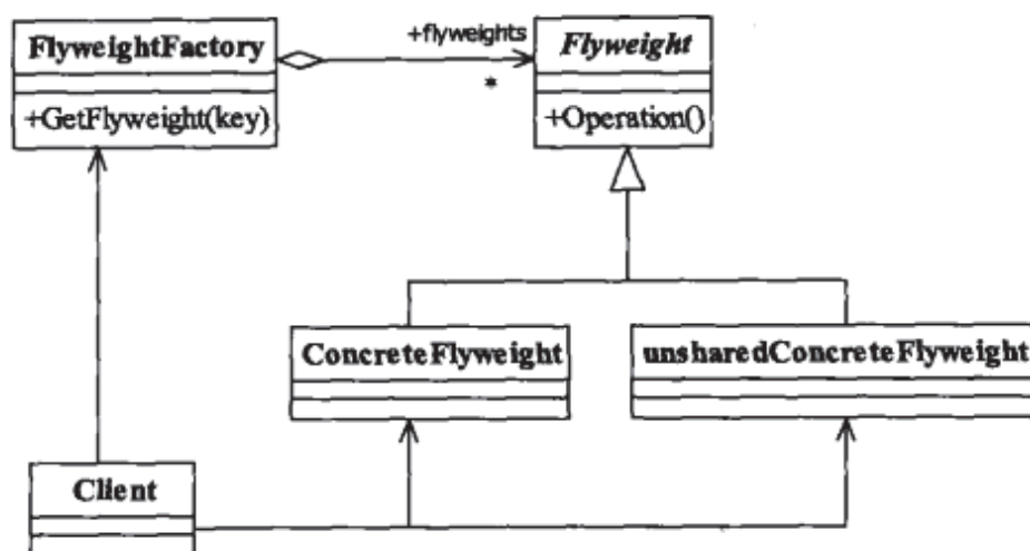
图28-3 享元模式的通用类图
