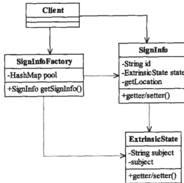
图28-4 类作为外部状态
