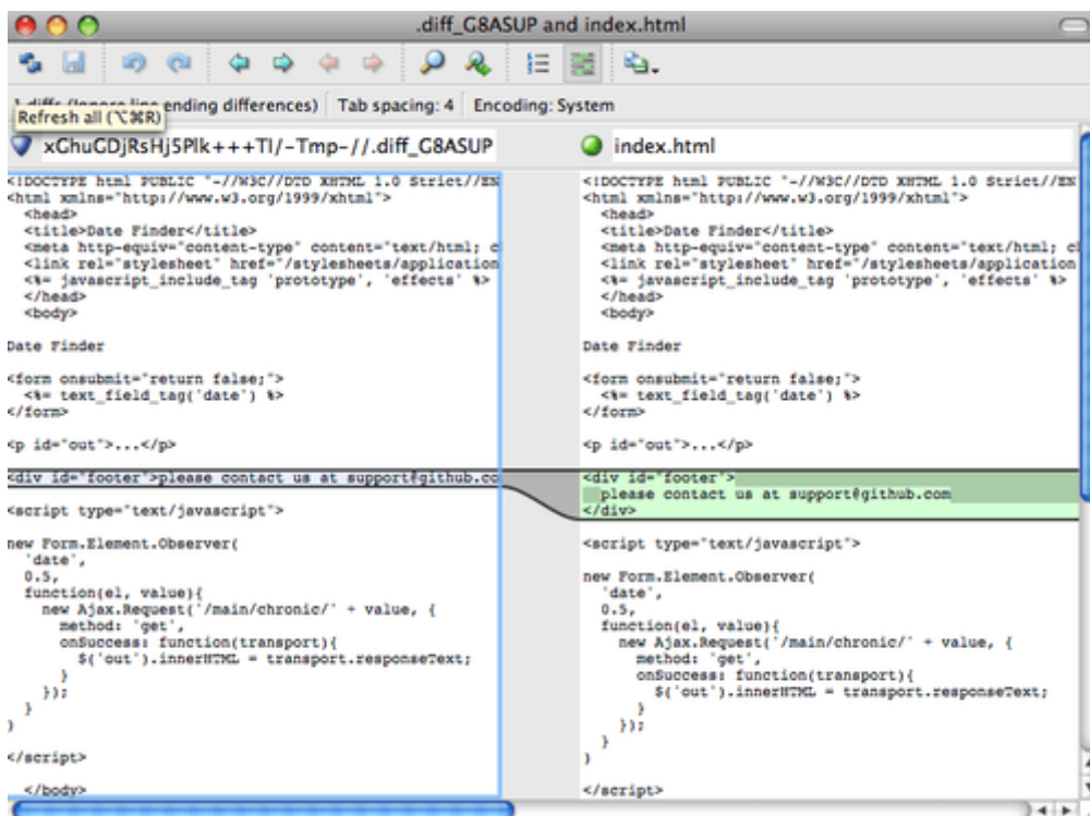
图 7-1. P4Merge.
